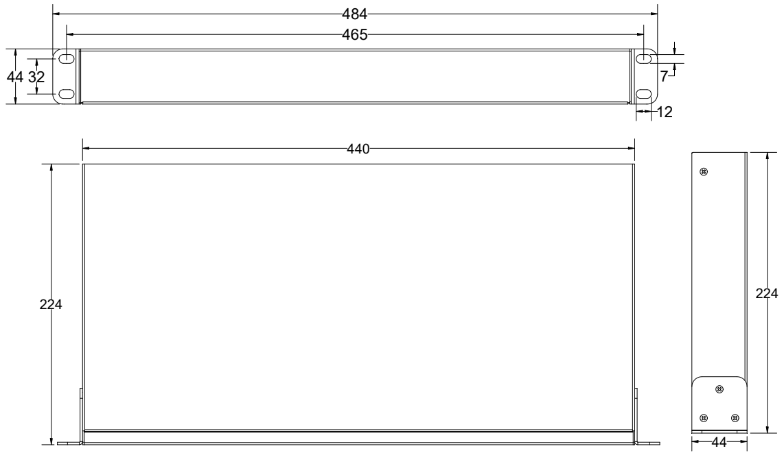
图 2.1 安装尺寸
