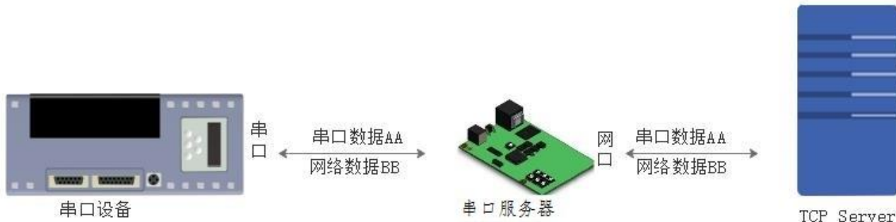
图 4.2 TCP Client 模式说明
