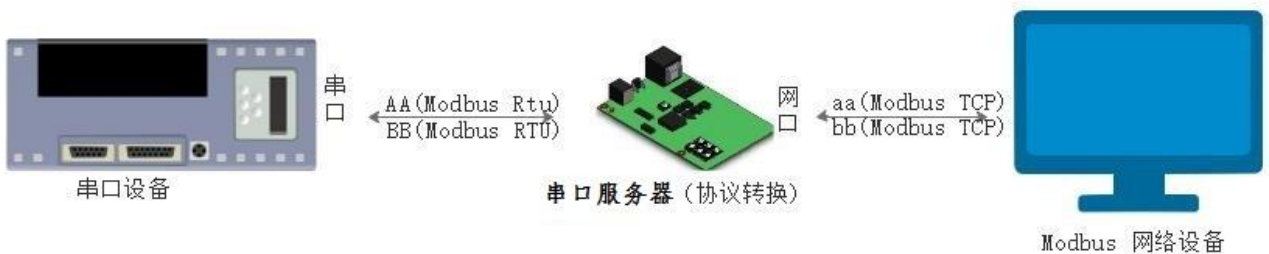
图 4.14 Modbus TCP
