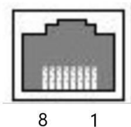
图 2.6 RJ45 插座接口定义
